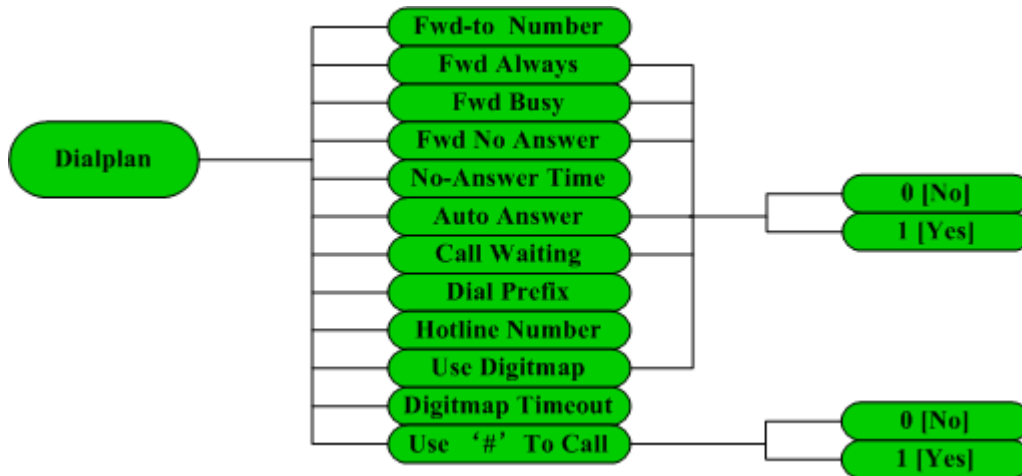
Fig 5.1.5 Dialplan submenu
